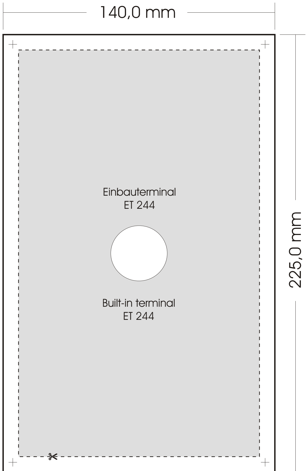
Einbauschablone für ET 244 Mounting diagram for ET 244
