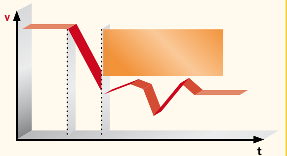
Sicher begrenzte Geschwindigkeit (Safety limited speed, SLS)
