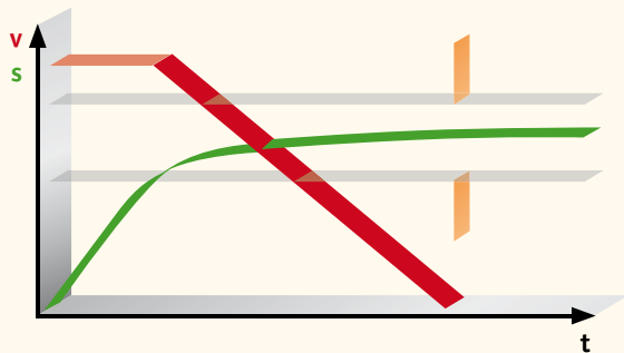
Sicherer Betriebsstopp (Safe operating stop, SOS)
