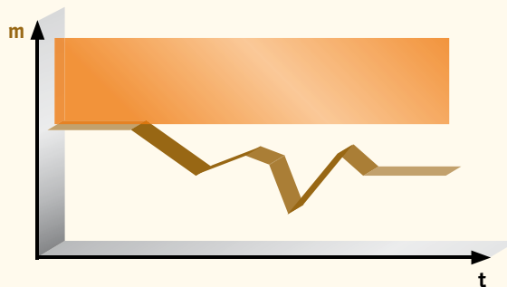
Sicher begrenztes Drehmoment (Safety limited torque, SLT)
