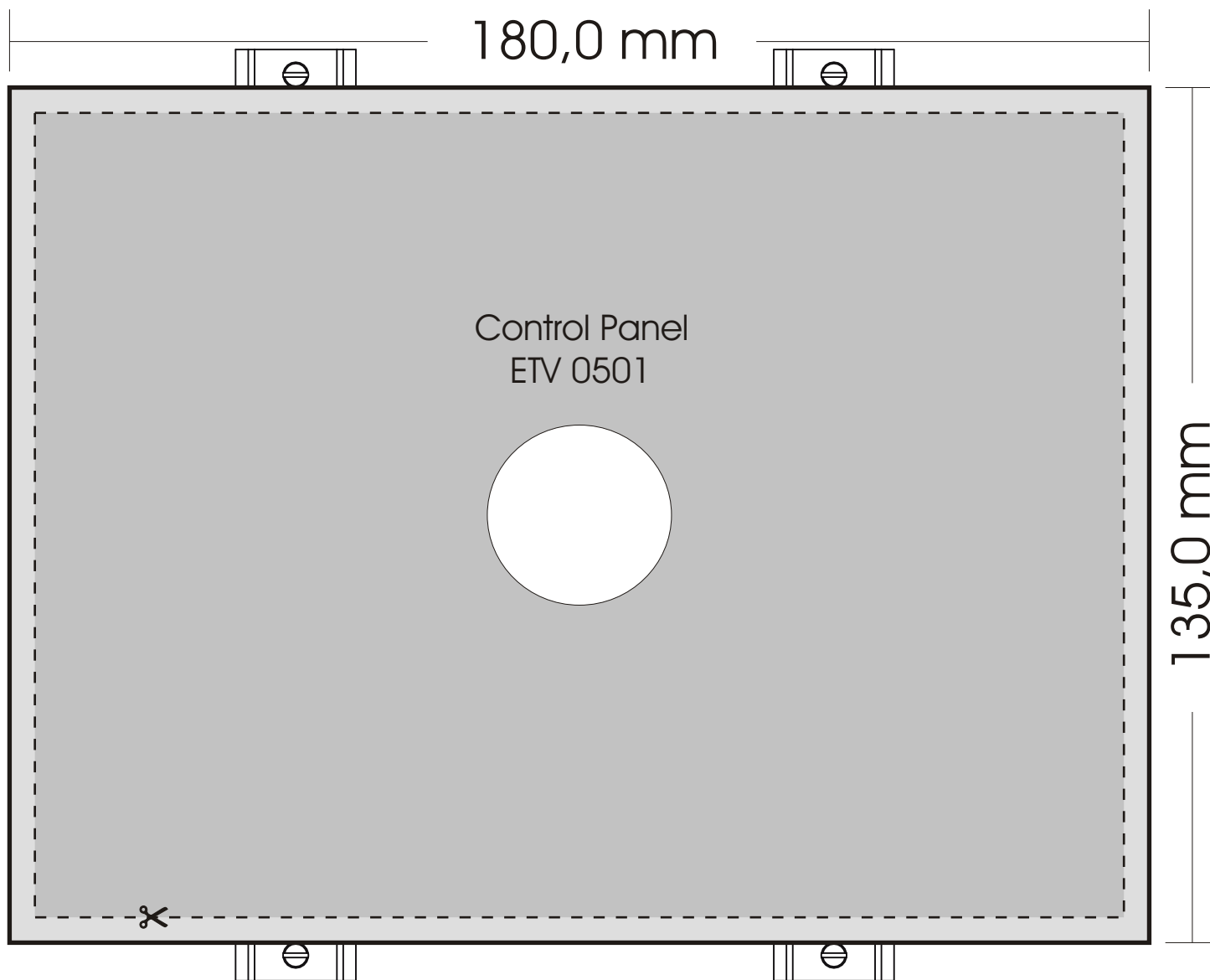
Einbauschablone für ETV 0501 Mounting diagram for ETV 0501
