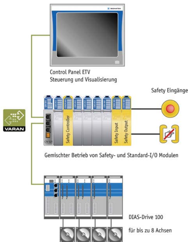
Bild 3: Wie das Beispiel einer Sigmatek-System-Architektur mit integrierter Safety zeigt, können die sicheren Ein- und Ausgangsmodule im Varan-Netzwerk beliebig verteilt angeordnet werden.
