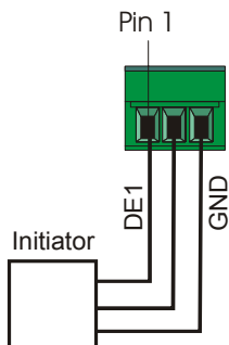
Anschlusschema 2
