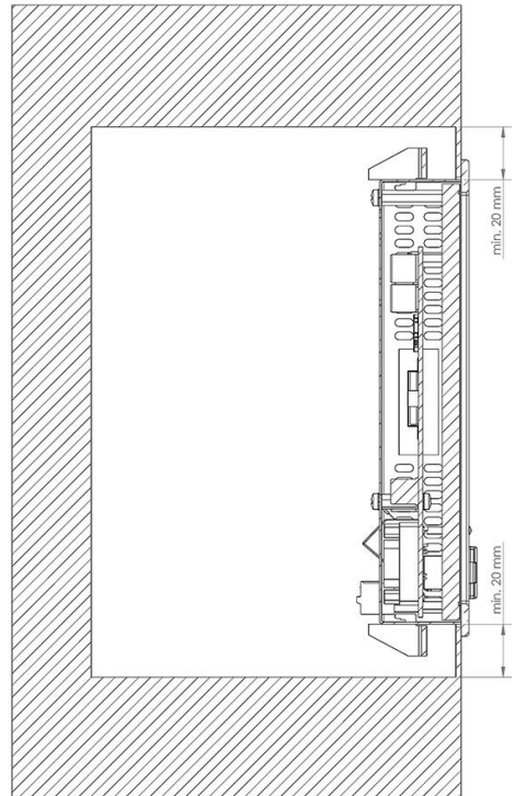
Schnitt Draufsicht:
