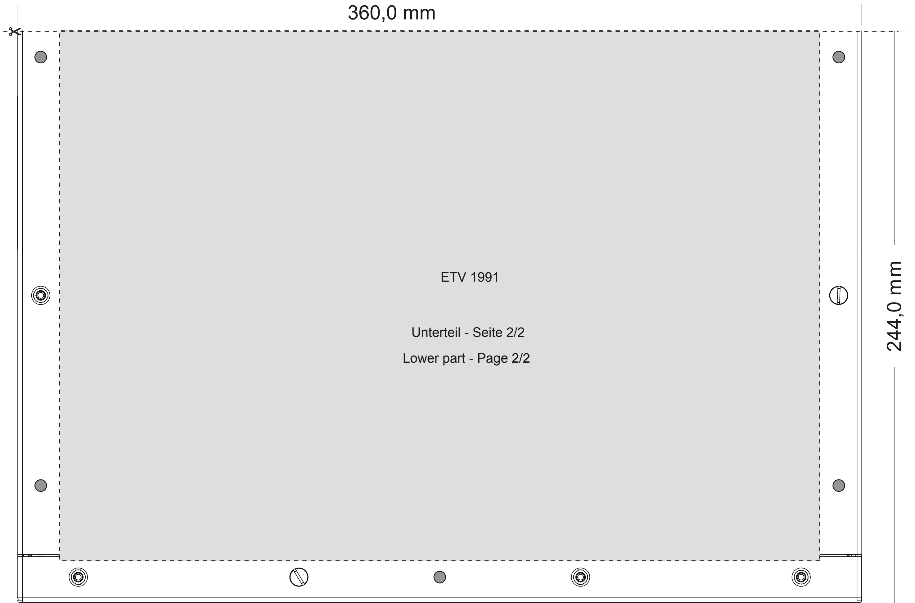
Einbauschablone für ETV 1991 Mounting diagram for ETV 1991
