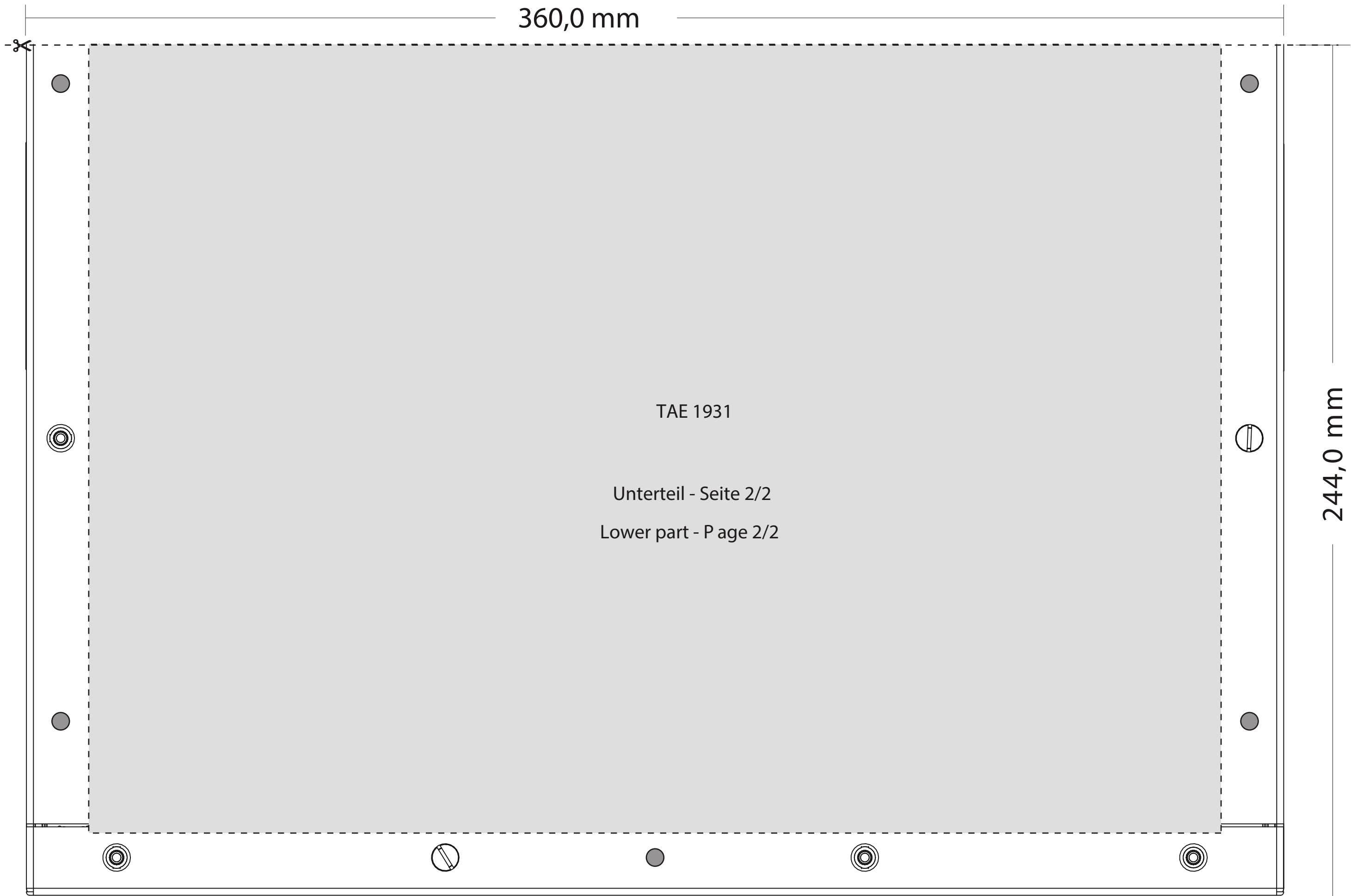
Einbauschablone für TAE 1931 Mounting diagram for TAE 1931
