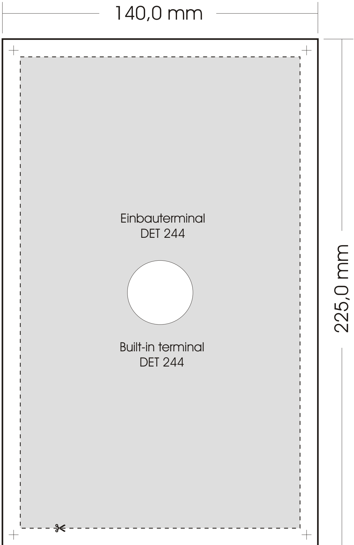
Einbauschaablone für DET 244 Mounting diagram for DET 244
