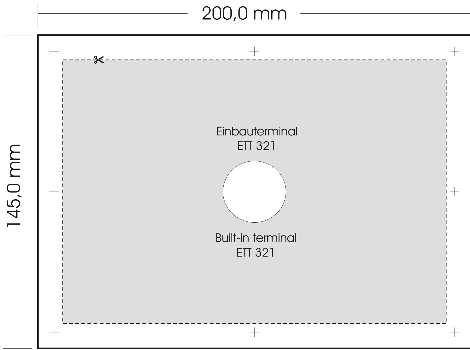
Einbauschaablone für ETT 321 Mounting diagram for ETT 321
