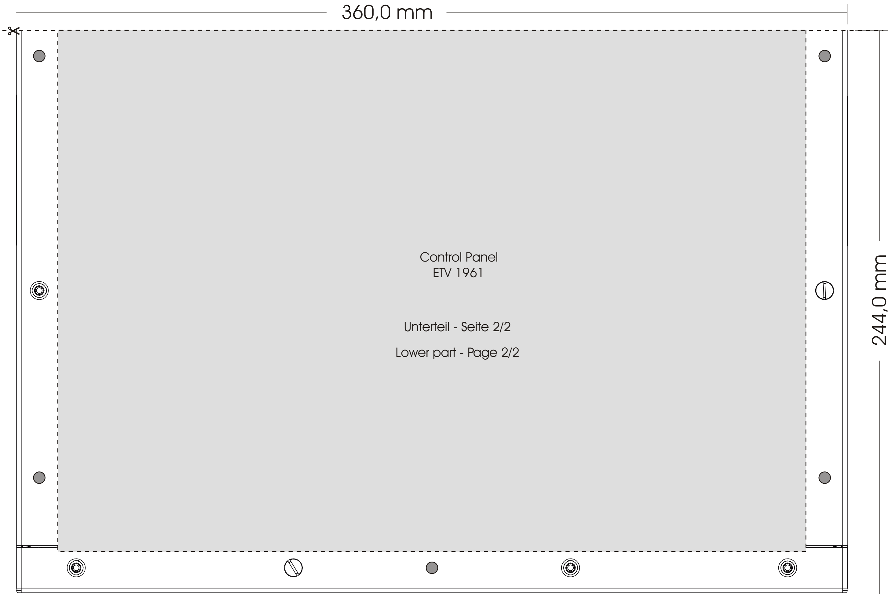
Einbauschablone für ETV 1961 Mounting diagram for ETV 1961
