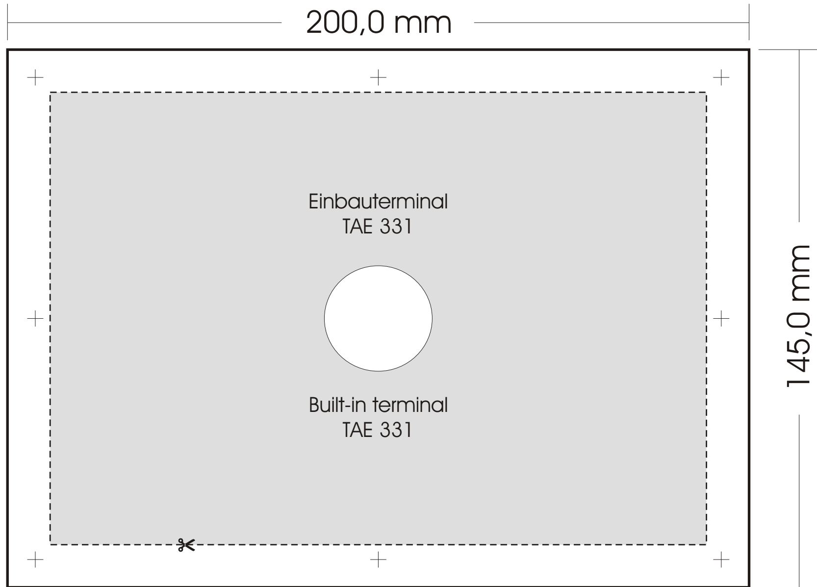
Einbauschablone für TAE 331 Mounting diagram for TAE 331
