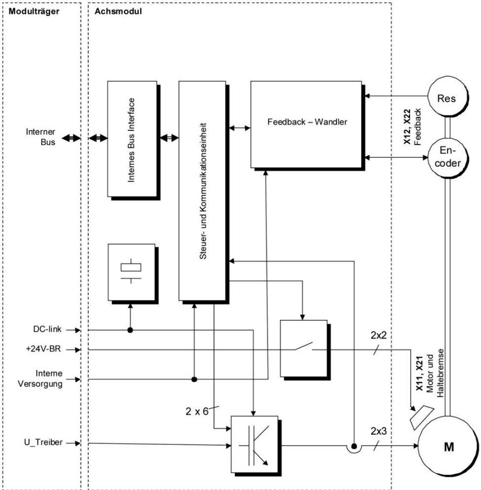
Blockschaltbild des Achsmoduls
