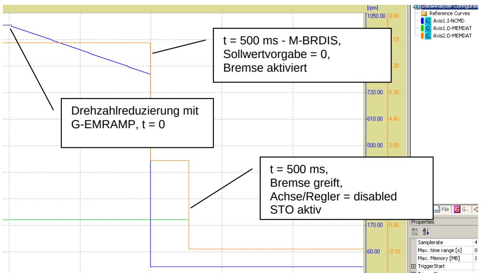
Zeitverhalten beim Öffnen des Sicherheitskreises
