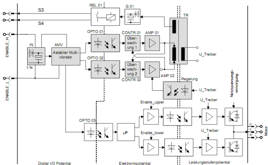
Blockschaltbild der sicheren Wiederanlaufsperrung
