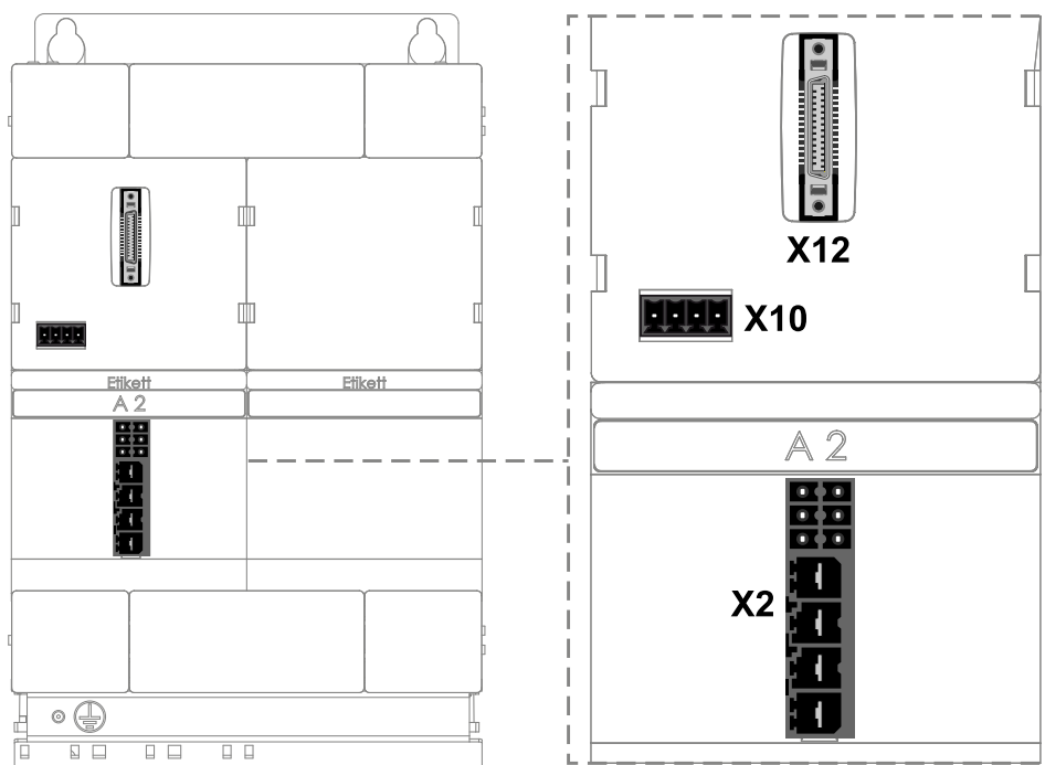
1-Achs-Gerät
