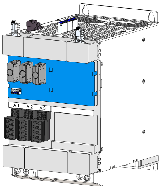
Baugröße 2
