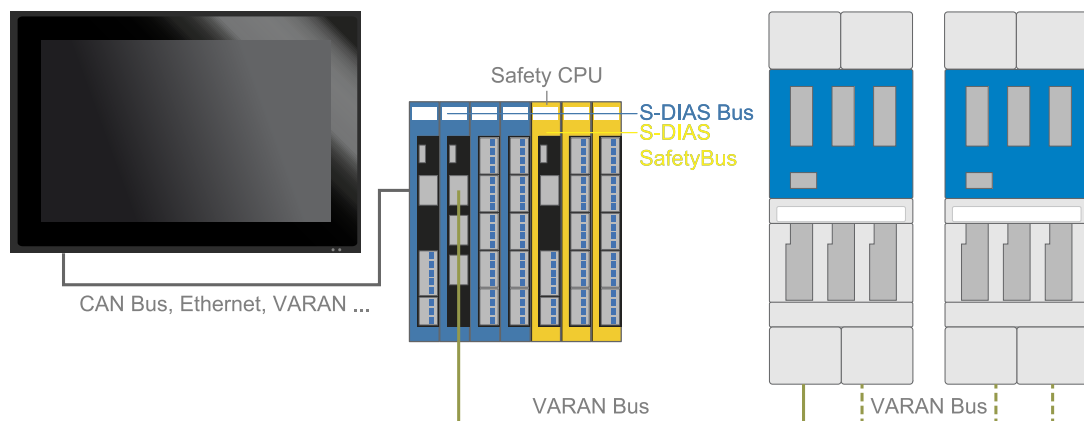
Beispiel Gesamtsystem
