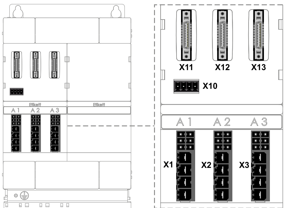
3-Achs-Gerät
