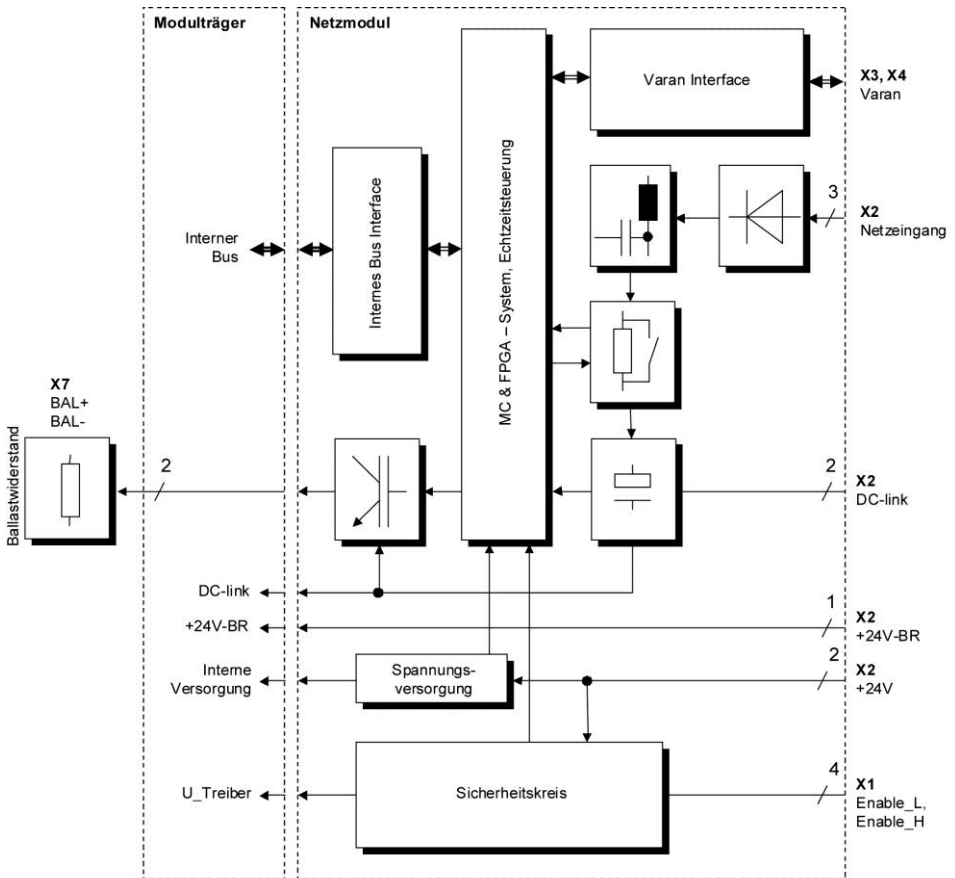
Blockschaltbild des Netzmoduls (Ballastwiderstand EXTERN )
