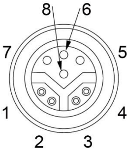
X1: Kabelanschluss M12 Y-Codiert
