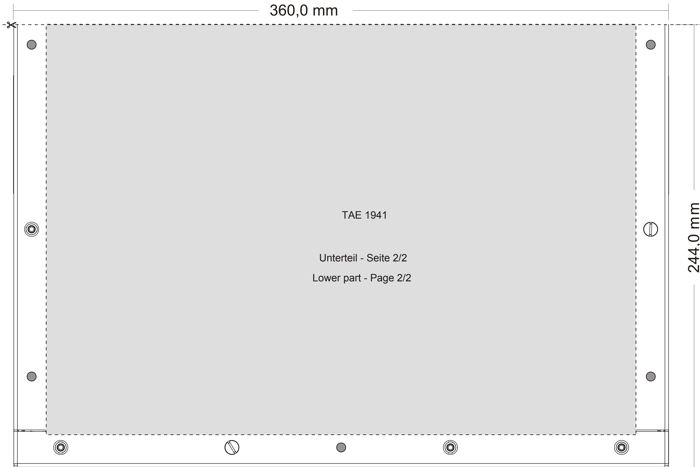
Einbauschablone für TAE 1941 Mounting diagram for TAE 1941
