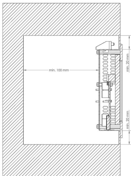
Schnitt Seitenansicht:
